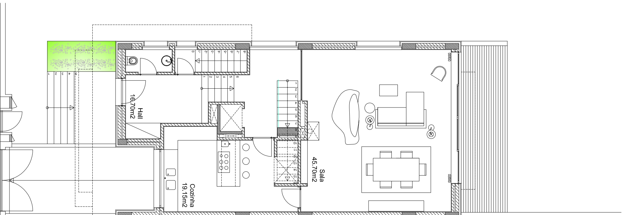
Planta do R/ch
