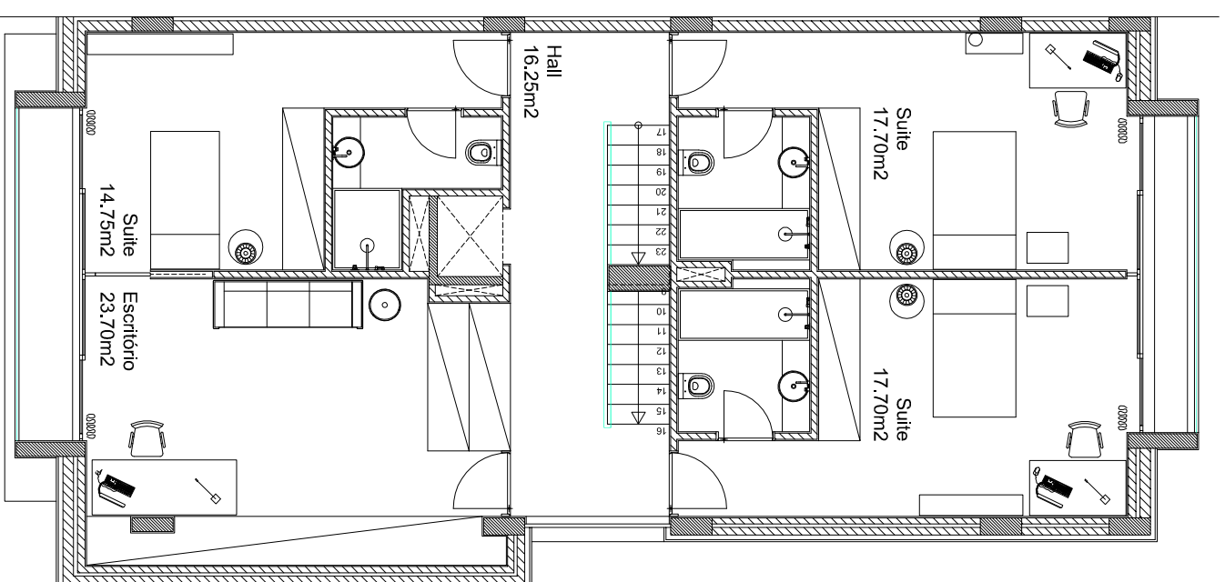
Planta do 1º Andar
