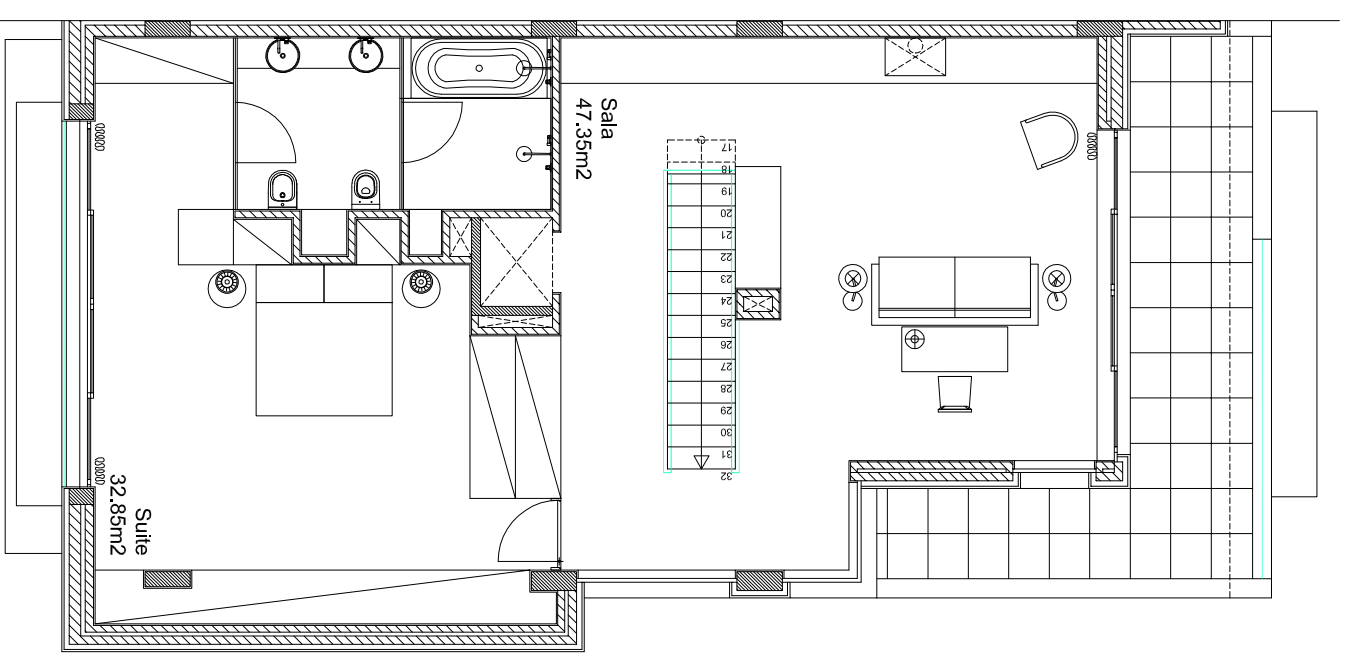
Planta do 2º Andar
