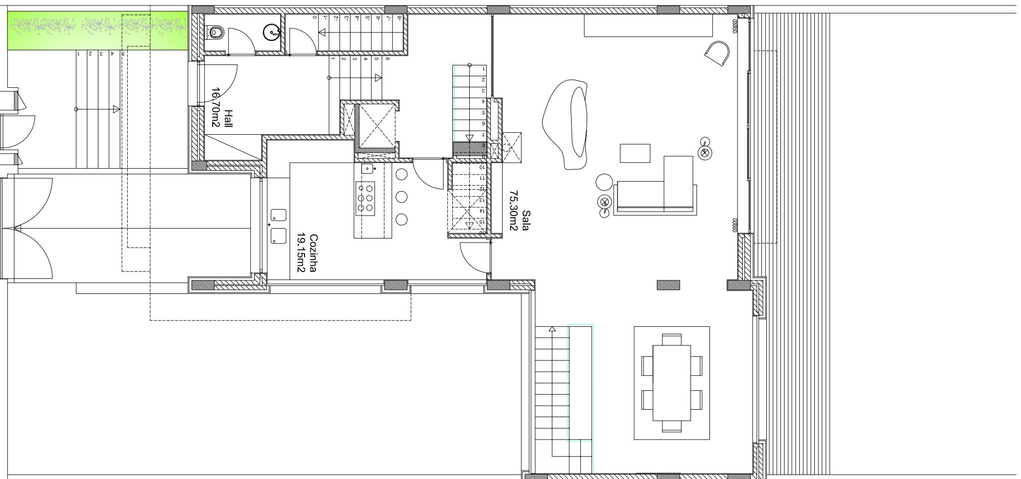
Planta do R/ch
